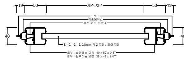
○ 세이프도어 평면도
