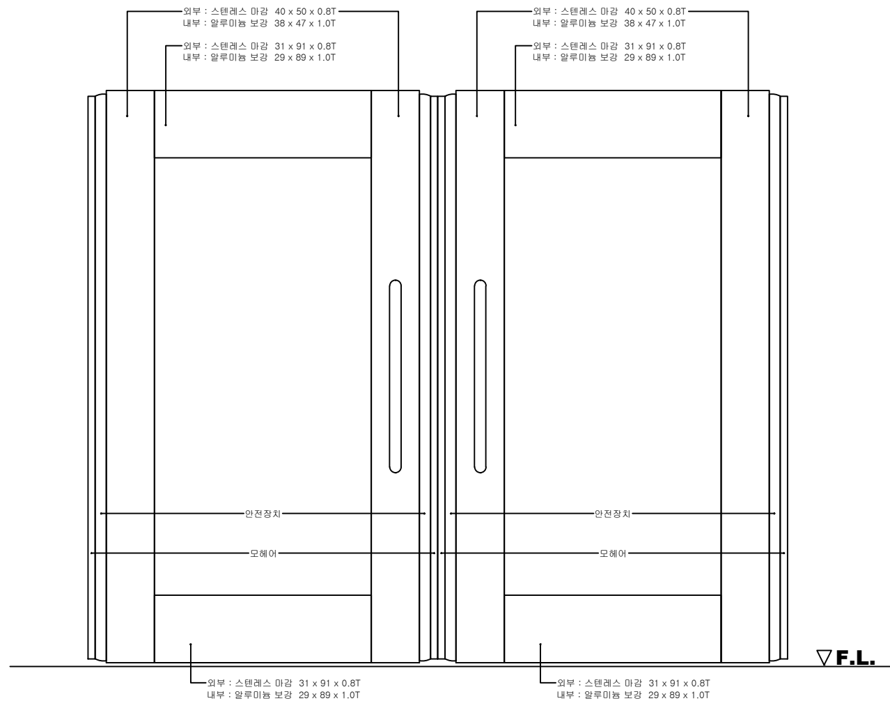
○ 세이프도어 정면도
