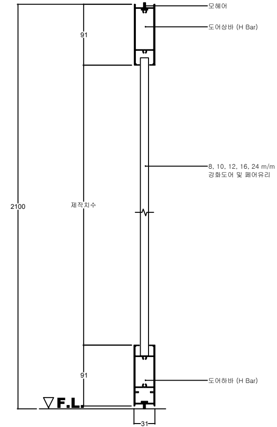
○ 세이프도어 측면도
