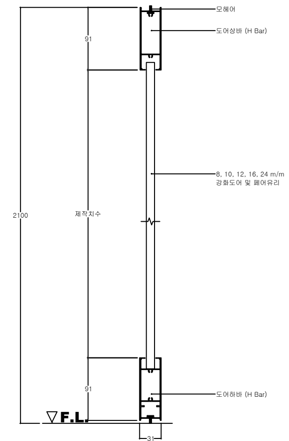
○ 세이프도어 측면도
