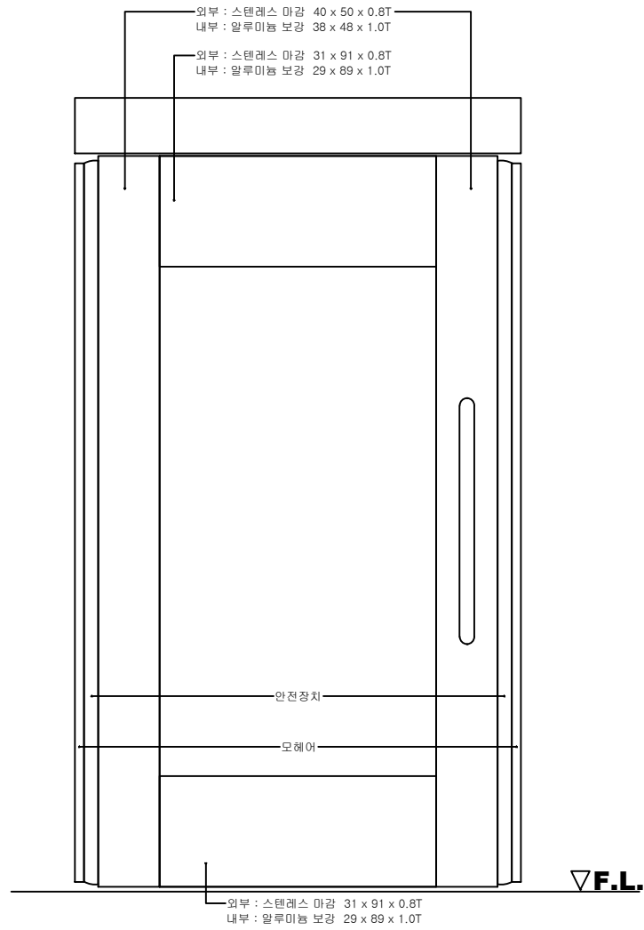
○ 세이프도어 정면도
